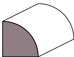
Quarto di tondo in Pino mm 20x20x3000
