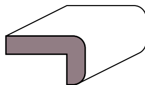
Terminale in Pino mm 26x20x3000 interno mm 20x10
