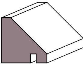
Gocciolatoio per infissi mm 25x25x3000
