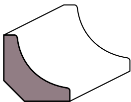
Angolare in Pino mm 28x13x3000
