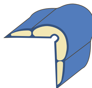
Coprispigolo antiurto PVC mm 35x35x1500
